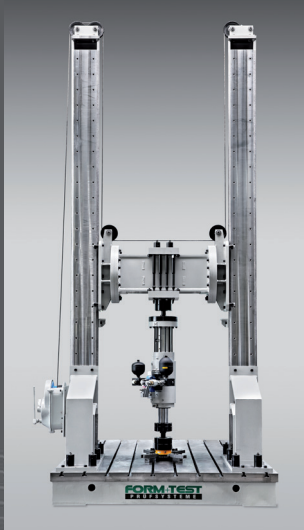
Prüfportal für stat. und dyn. Anwendungen im Automobilsektor
