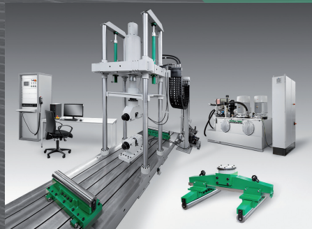
Statische und dynamische Zug-, Druck- und Biegeprüfungen an großen Bauteilen
